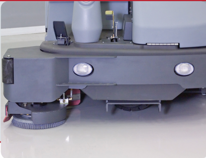
ER 1600 (right scrub unit)
